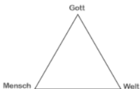
Abbildung 1: Das "Dreiecksproblem"
